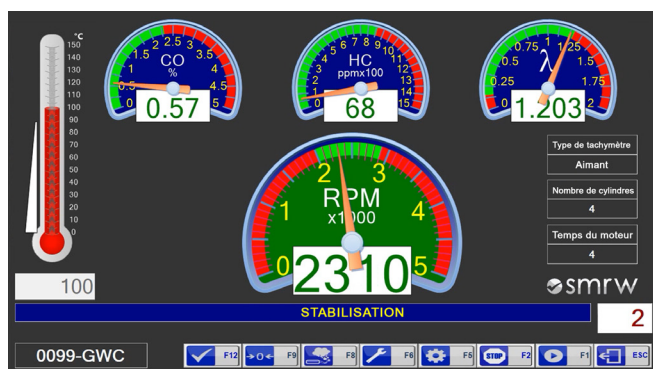
LOGICIEL ANALYSEUR DE GAZ RY-4000AH
